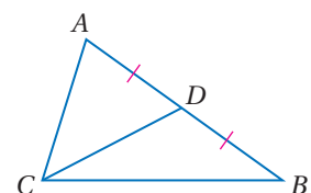
\overline{CD} قطع متوسطة في \triangle ABC .
