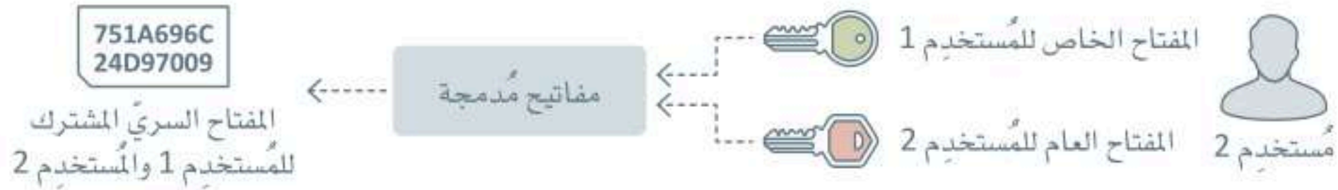
شكل 3.9: تمثيل خوارزمية ديفي-هيلمان لتبادل المفاتيح
