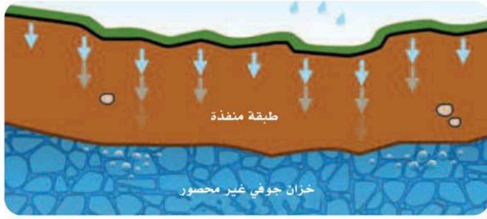
الشكل 17-6 طبقة غير محصورة.
