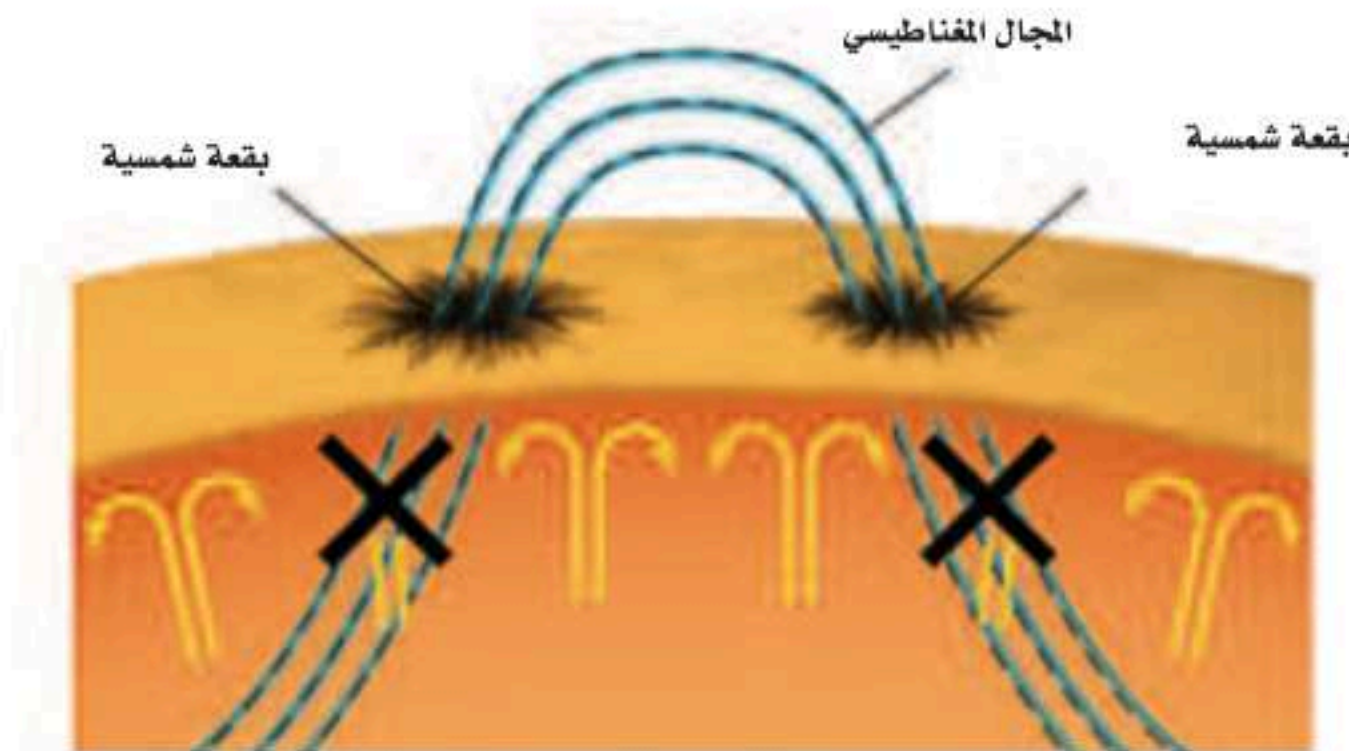
الشكل 7-2 التواء خطوط المجال المغناطيسي بسبب الدوران التفاضلي للشمس ونشوء البقع الشمسية.
