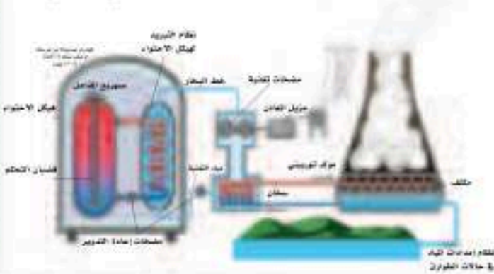
مفاعل ماء - مغلي نموذجي
