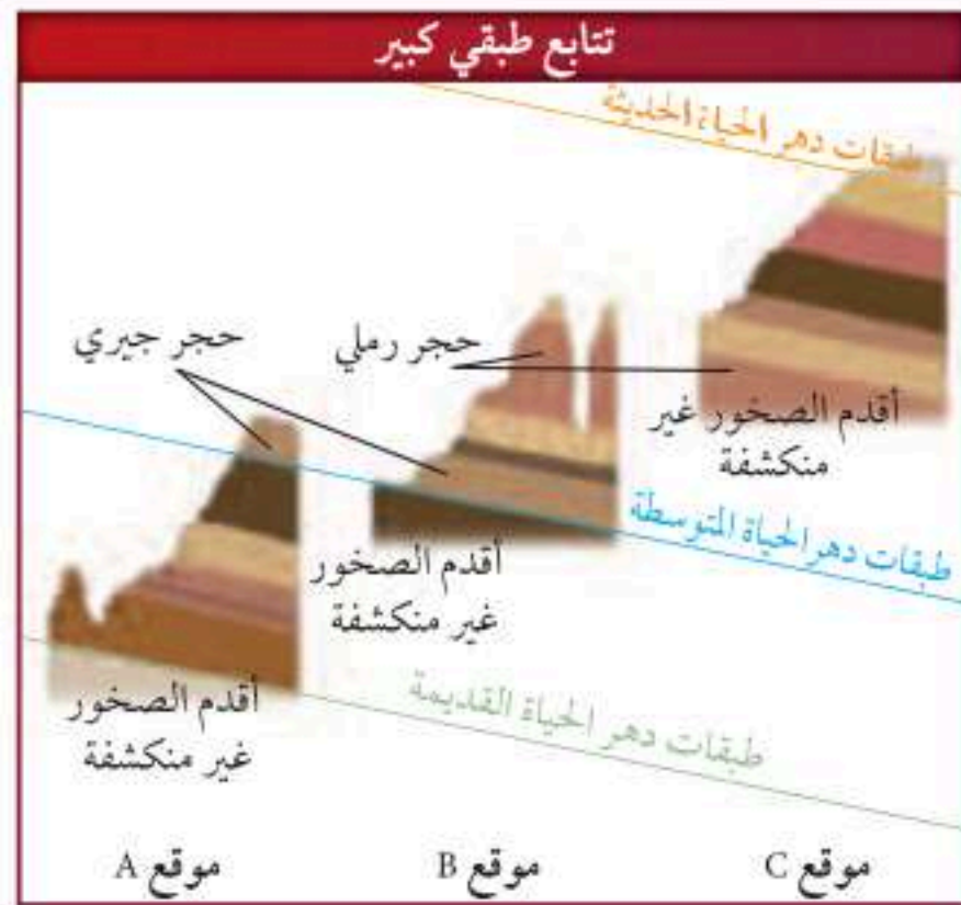
الشكل 23-4 يمثل الحجر الجيري أحدث الطبقات الصخرية في الموقع A وأقدمها في الموقع B، وطبقة الحجر الرملي تمثل أحدث الطبقات الصخرية في الموقع B ولكنها تعد صخوراً غير منكشفة في الموقع C. استنتج تركيب الطبقة المدفونة أسفل طبقة الحجر الجيري عند الموقع B.
