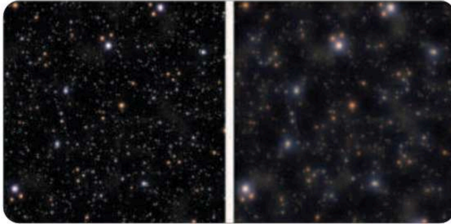
الشكل 8-3 صورة توضح الزيغ الكروي.
